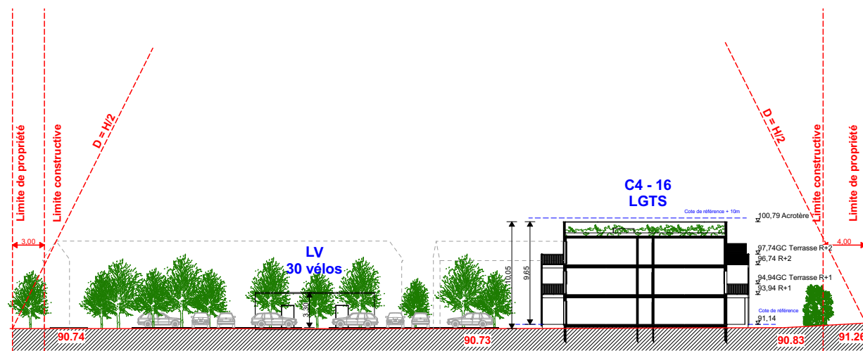
COUPE B'-B'
